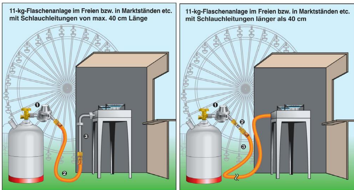
11-kg-Flaschenanlage im Freien bzw. in Marktständen etc. mit Schlauchleitungen von max. 40 cm Länge
